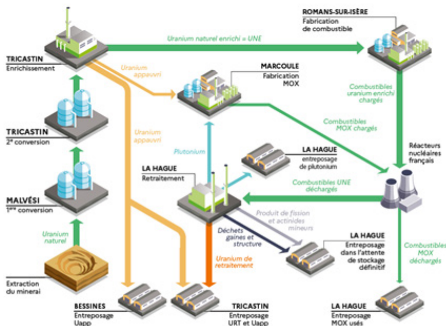
Figure 32. Les installations françaises du cycle du combustible nucléaire en 2024
