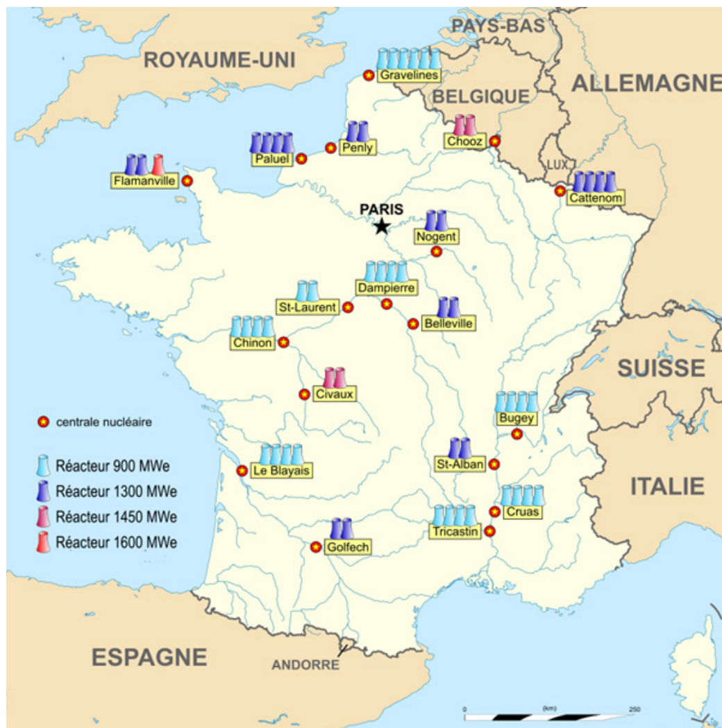
Figure 30. Les réacteurs électronucléaires français en fonctionnement en 2024
